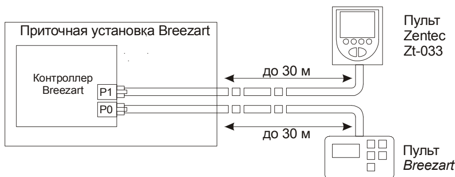
Рисунок 1.9 Подключение пульта Zentec Zt-033
