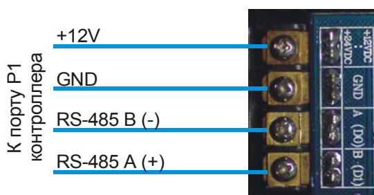
Рисунок 1.10 Схема подключения цепей порта P1 к пульту Zentec Zt-033
