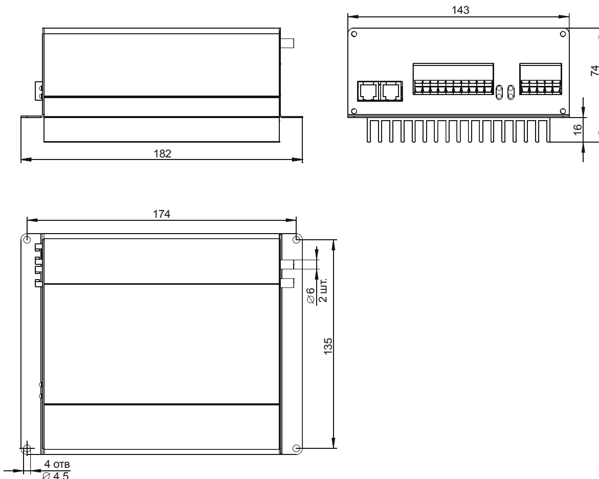
Рисунок 1.3 - Габаритный чертёж контроллера
