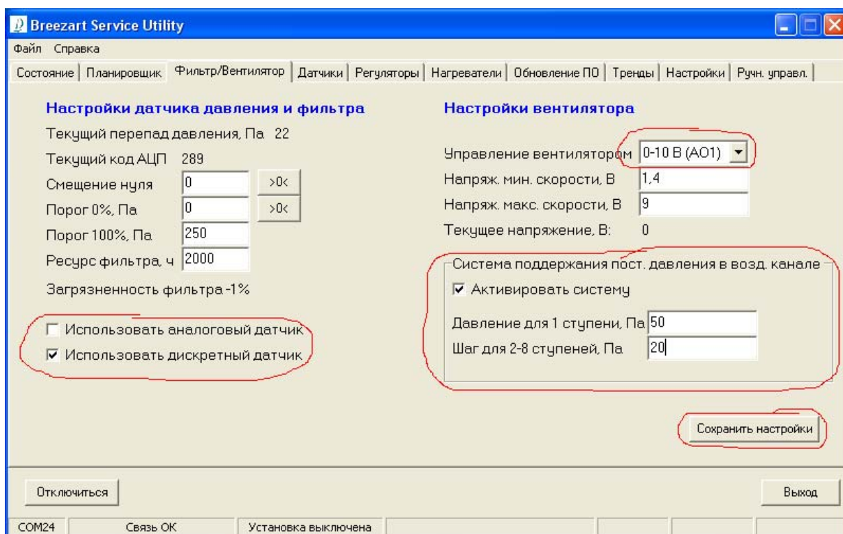
Рисунок 1.12 - Настройка VAV-системы
